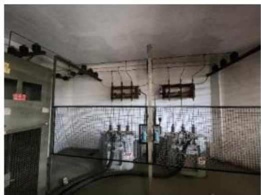
Figura 15 – Transformadores na SE.
